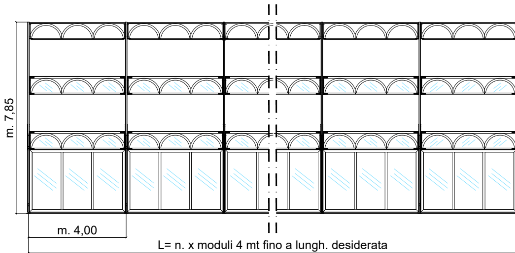
PROSPETTO LATERALE
